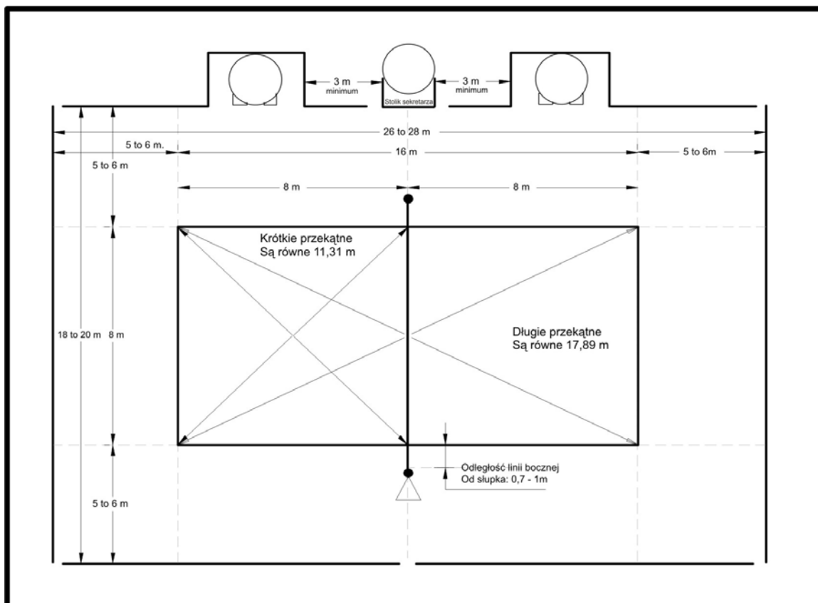
Rzut boiska - Rys. 1
